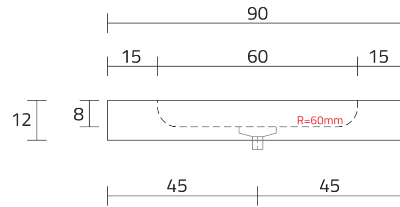
ROZMIESZCZENIE ODPŁYWU
