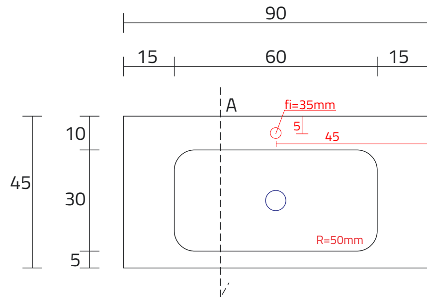
RZUT Z GÓRY
