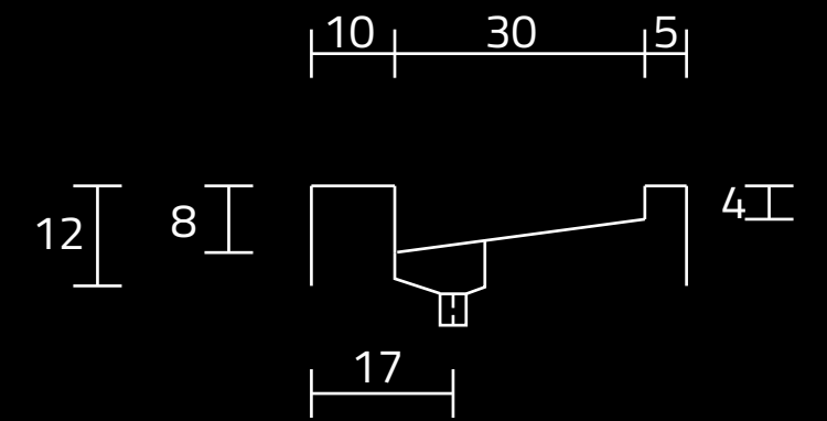
PRZEKRÓJ ,A'
