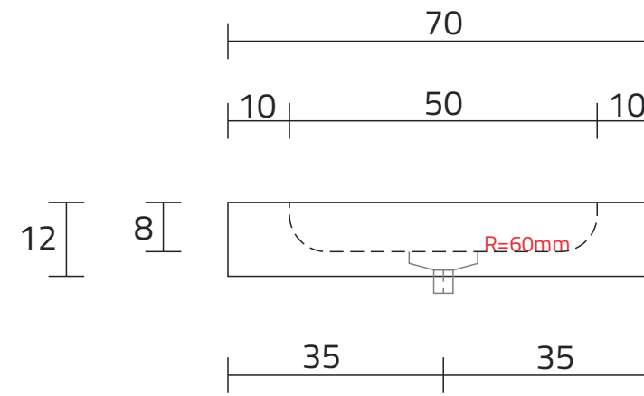
ROZMIESZCZENIE ODPŁYWU
