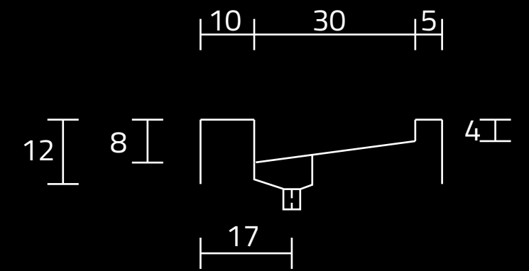
PRZEKRÓJ ,A'
