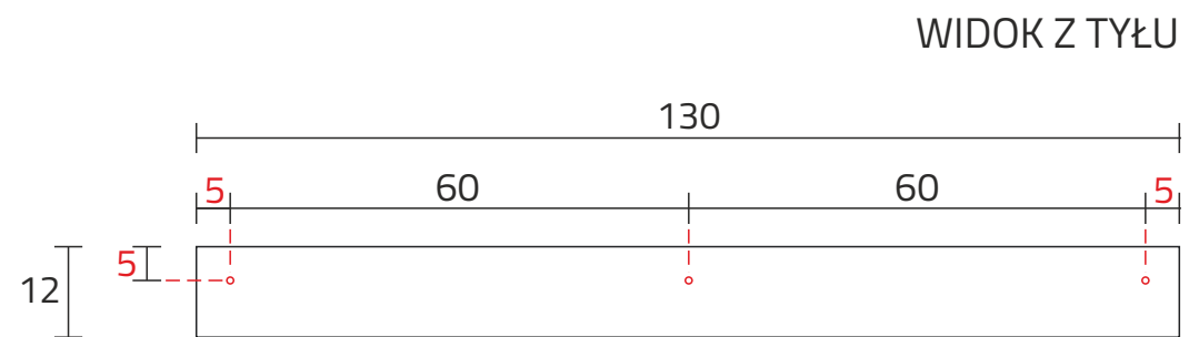
OTWORY MONTAŻOWE
