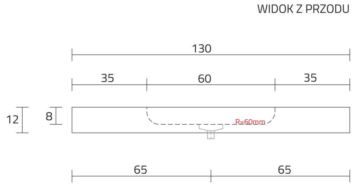
ROZMIESZCZENIE ODPŁYWU
