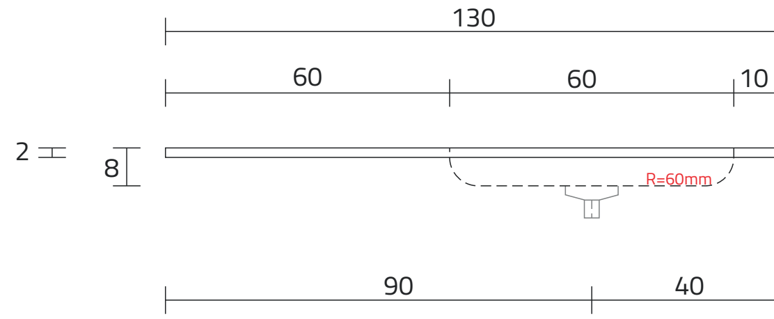
ROZMIESZCZENIE ODPŁYWU
