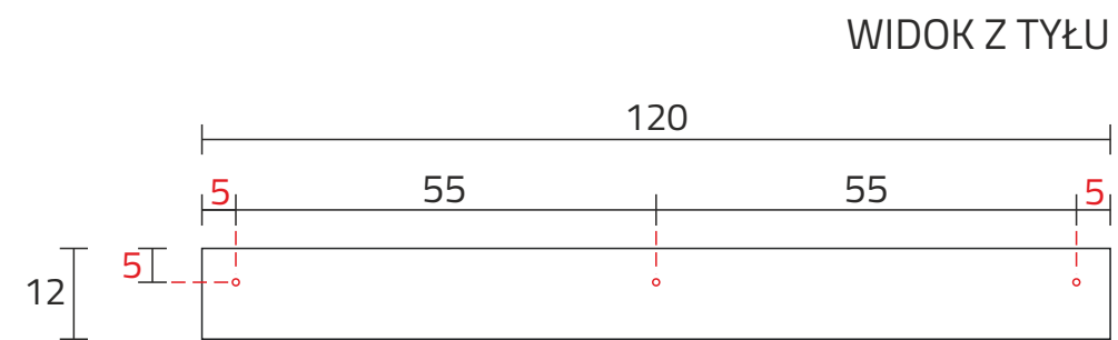
OTWORY MONTAŻOWE
