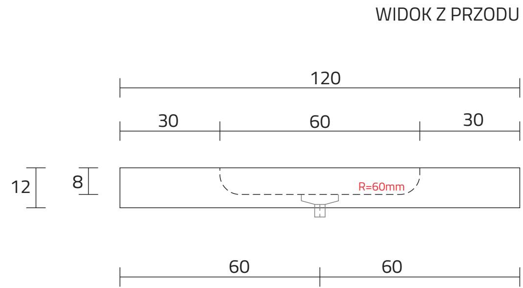
ROZMIESZCZENIE ODPŁYWU
