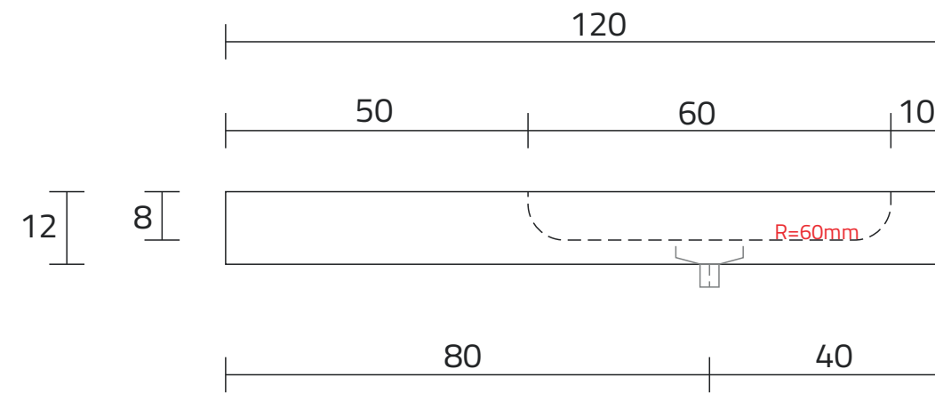
ROZMIESZCZENIE ODPŁYWU
