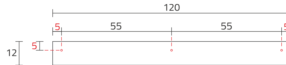
OTWORY MONTAŻOWE
