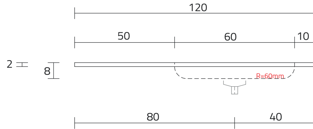
ROZMIESZCZENIE ODPŁYWU
