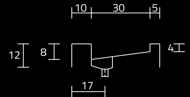
PRZEKRÓJ ,A'
