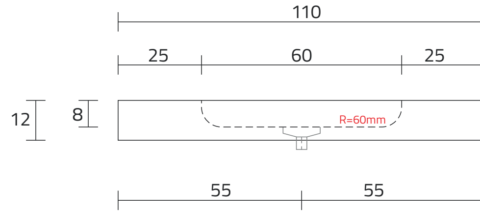
ROZMIESZCZENIE ODPŁYWU
