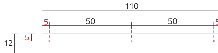
OTWORY MONTAŻOWE
