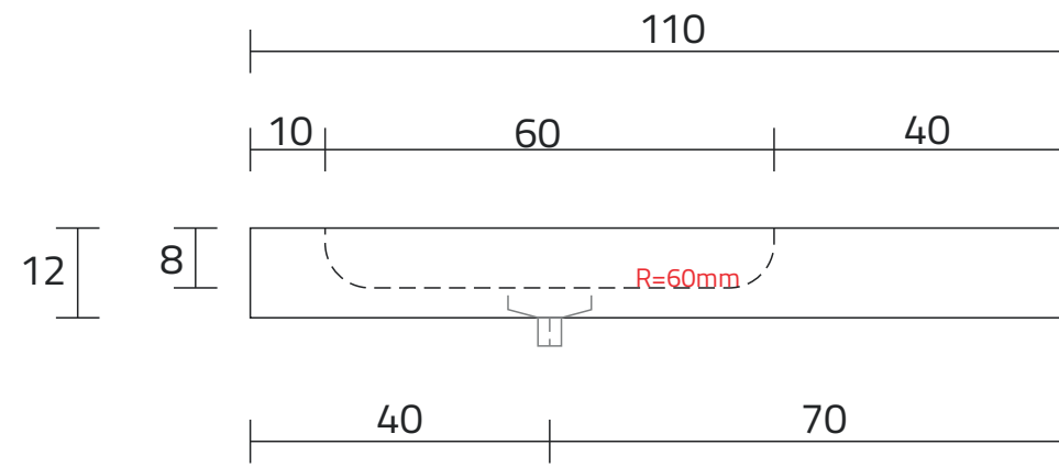
ROZMIESZCZENIE ODPŁYWU
