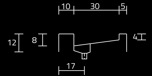
PRZEKRÓJ ,A'
