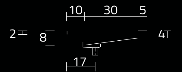
PRZEKRÓJ ,A'
