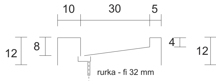
PRZEKRÓJ
